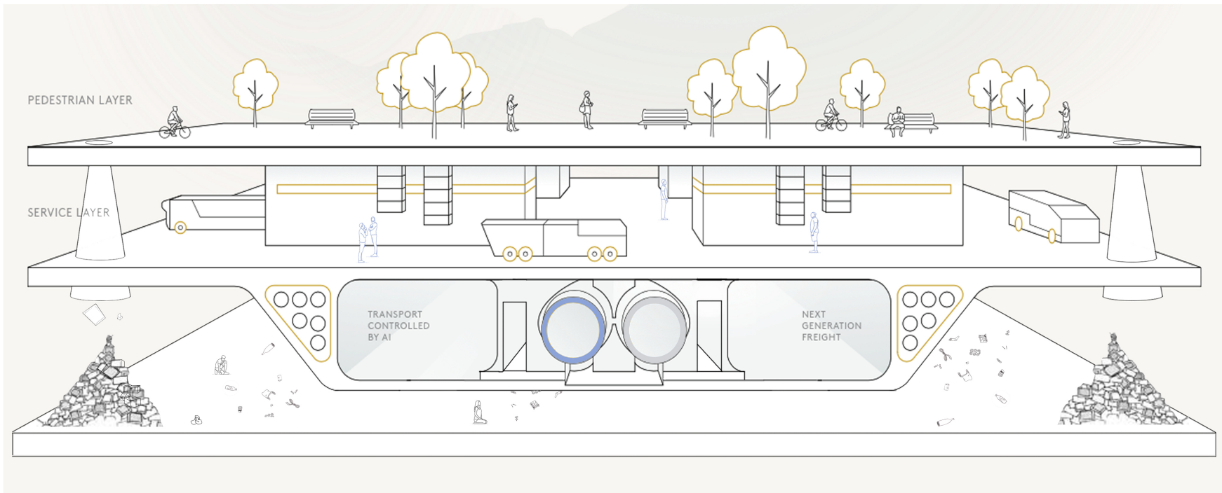
COUPE TRANSVERSALE ESPACES SOUTERRAINS
