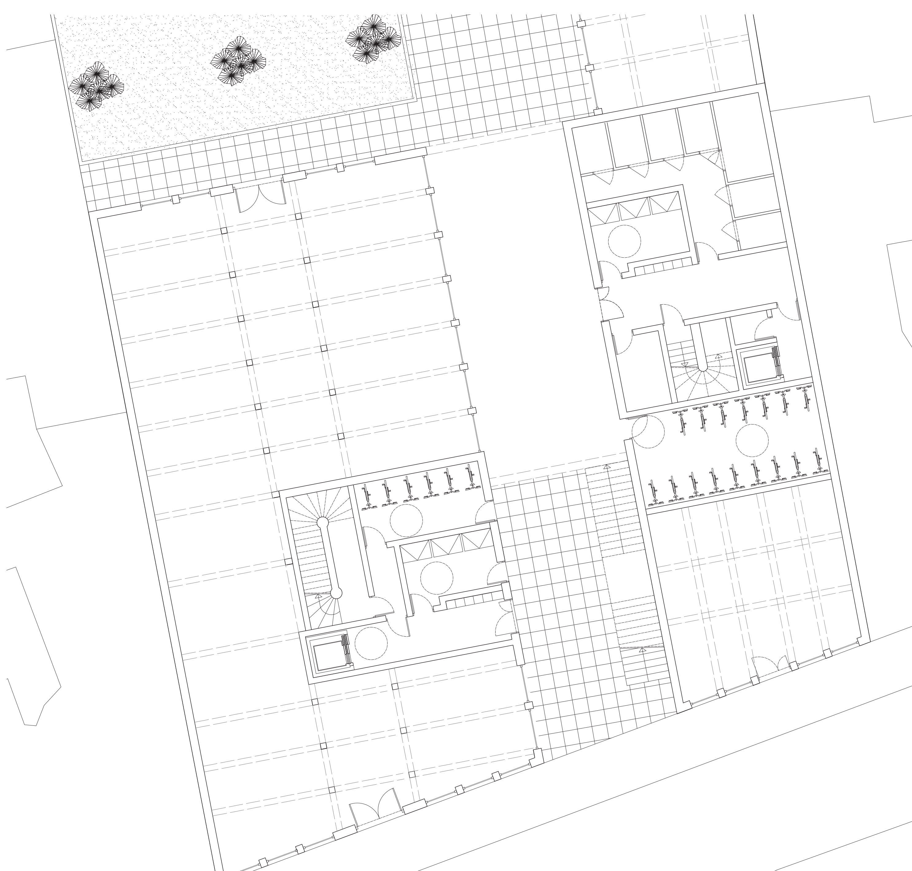
PLAN RDC
