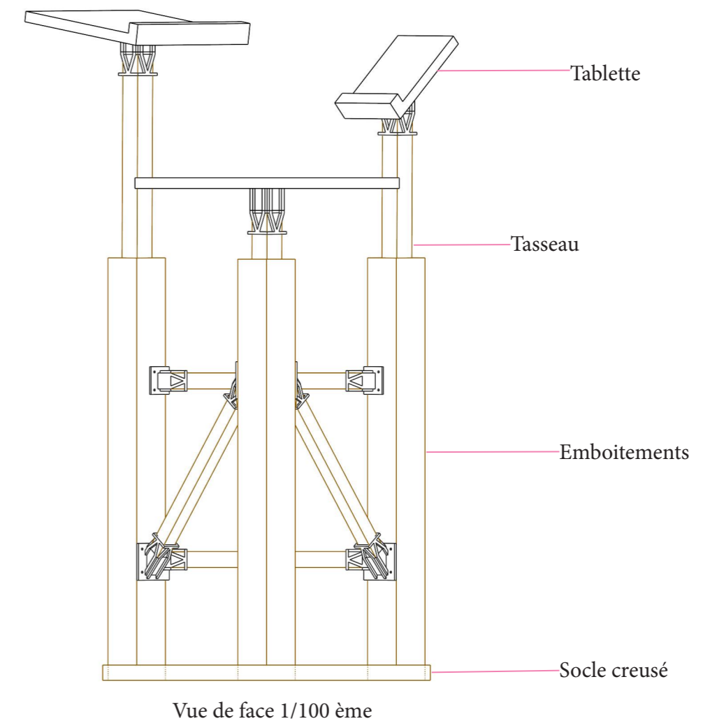
Vue de face 1/100ème
