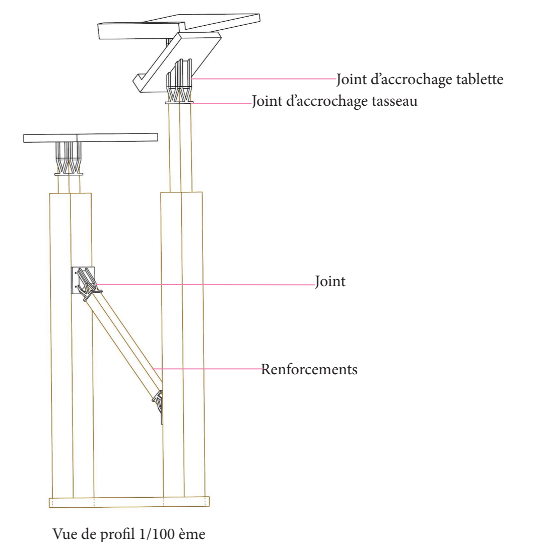
Vue de profil 1/100ème
