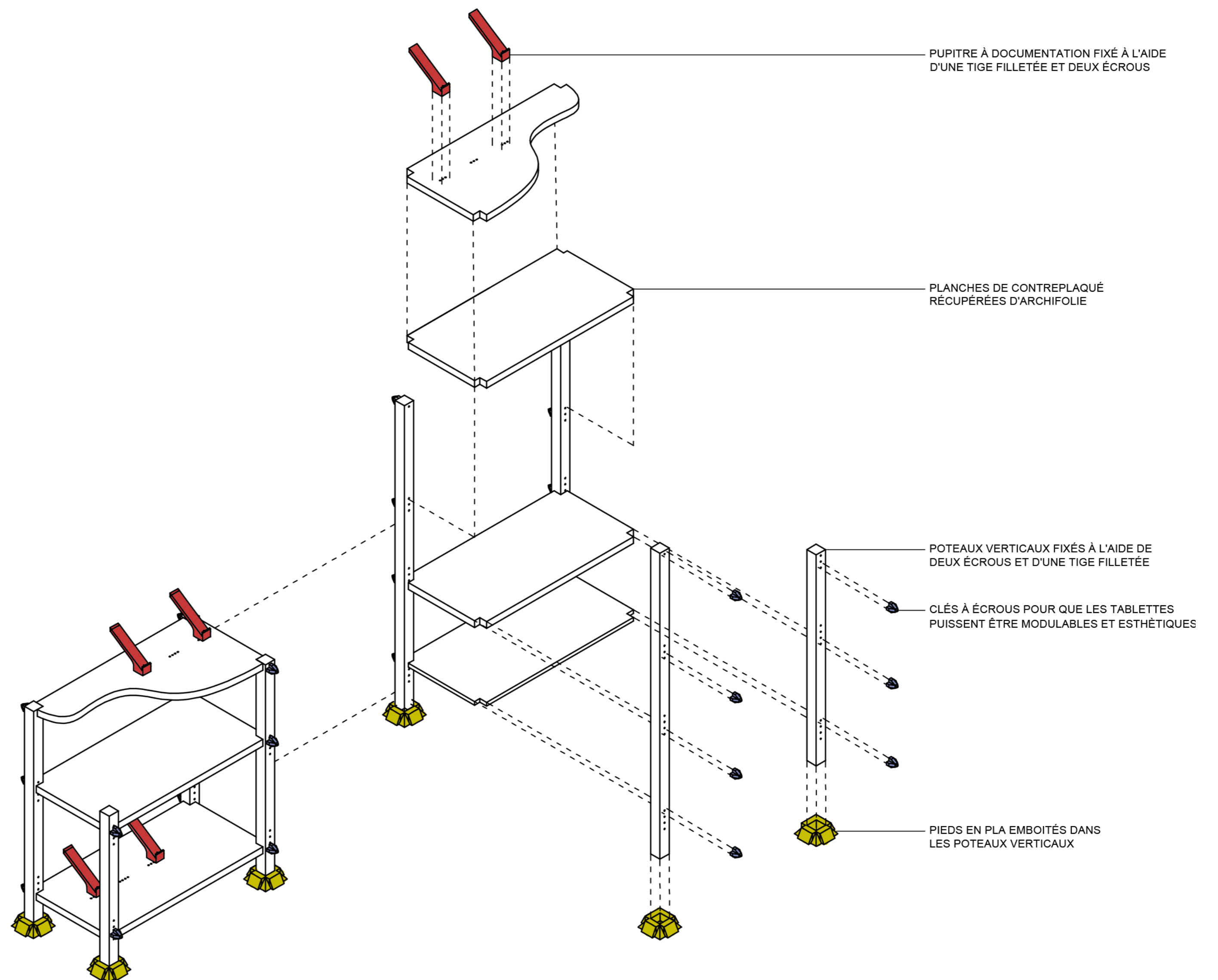
Axonométrie
