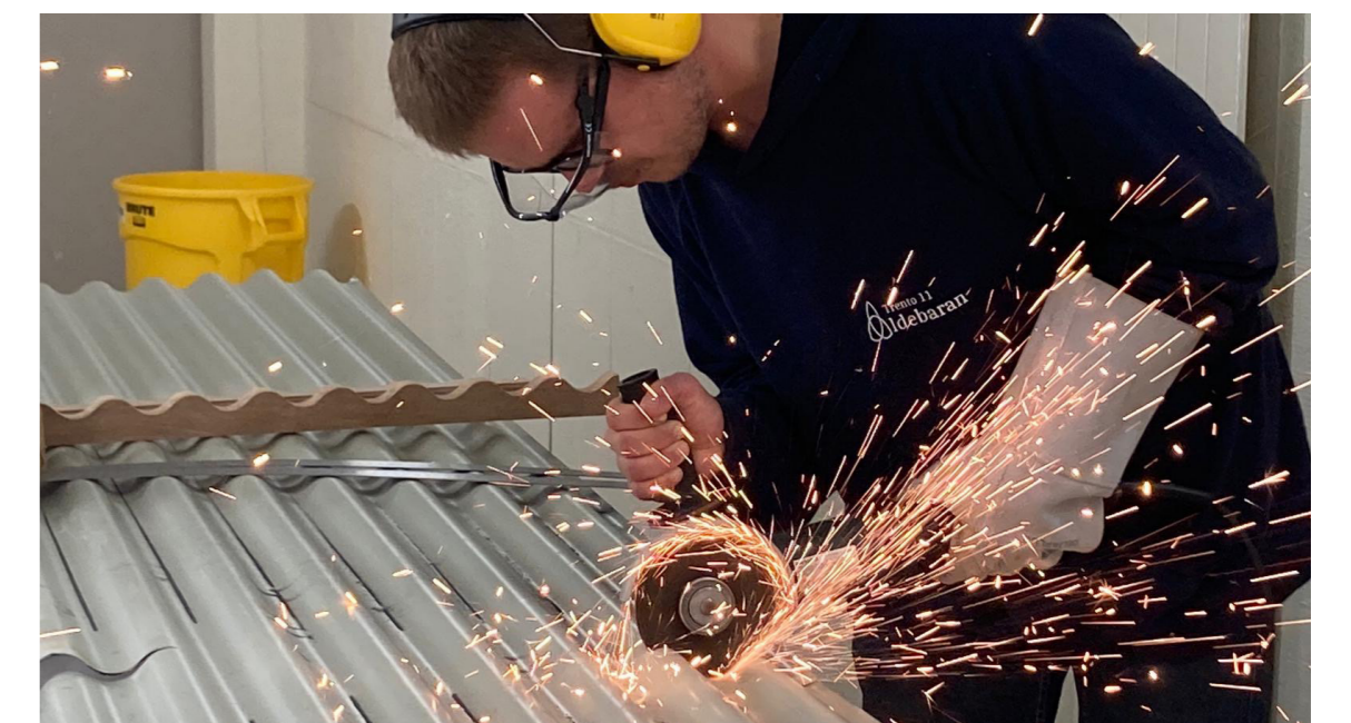
Découpe de la tôle
