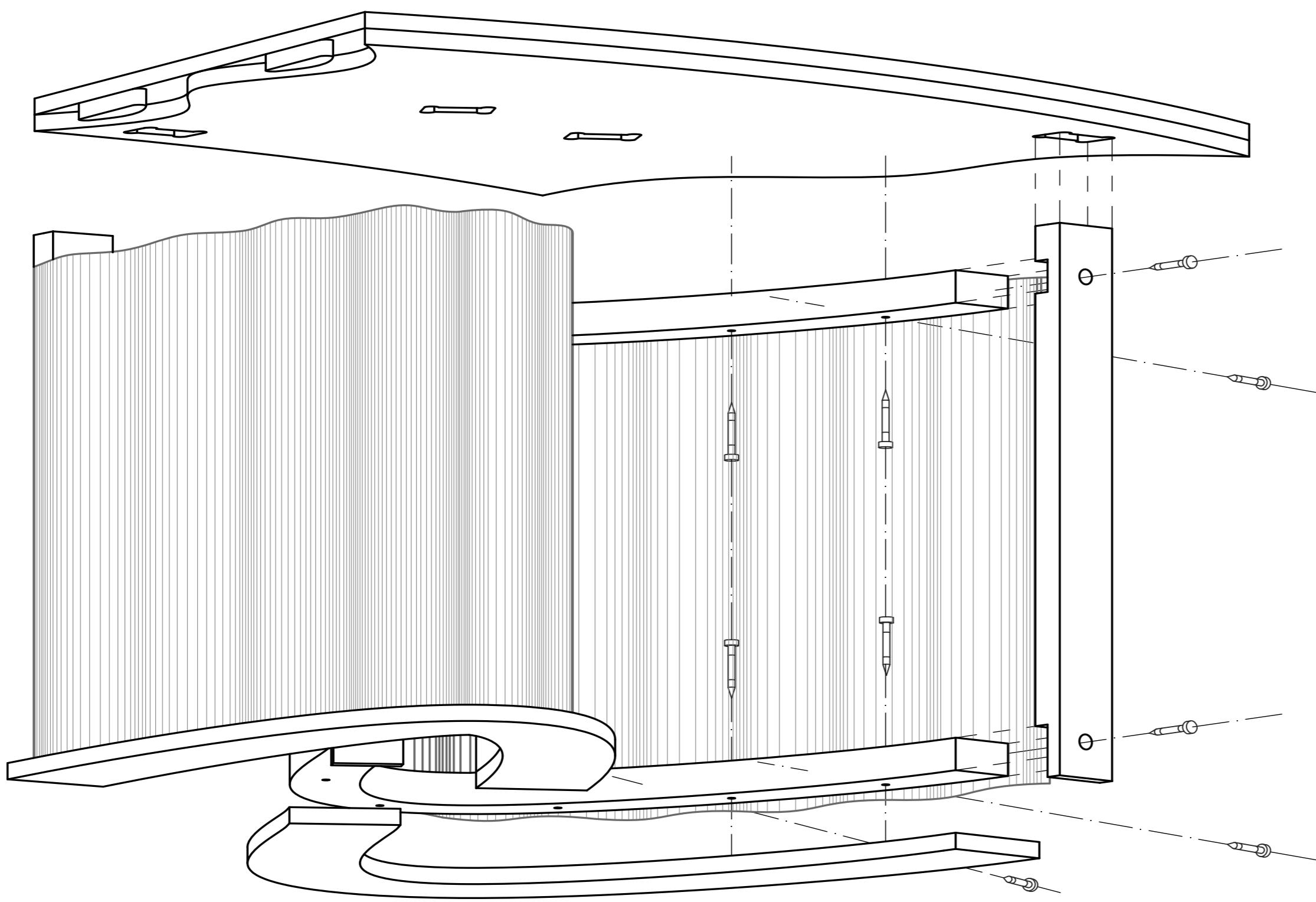
Axonométrie éclatée Assemblages
